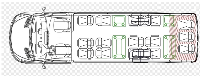
Приложение 2 - Сиденья - Расположение сидений
